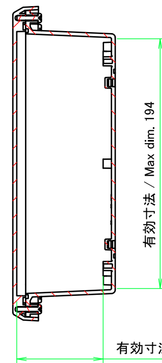
A-A ( 1 : 3 )
